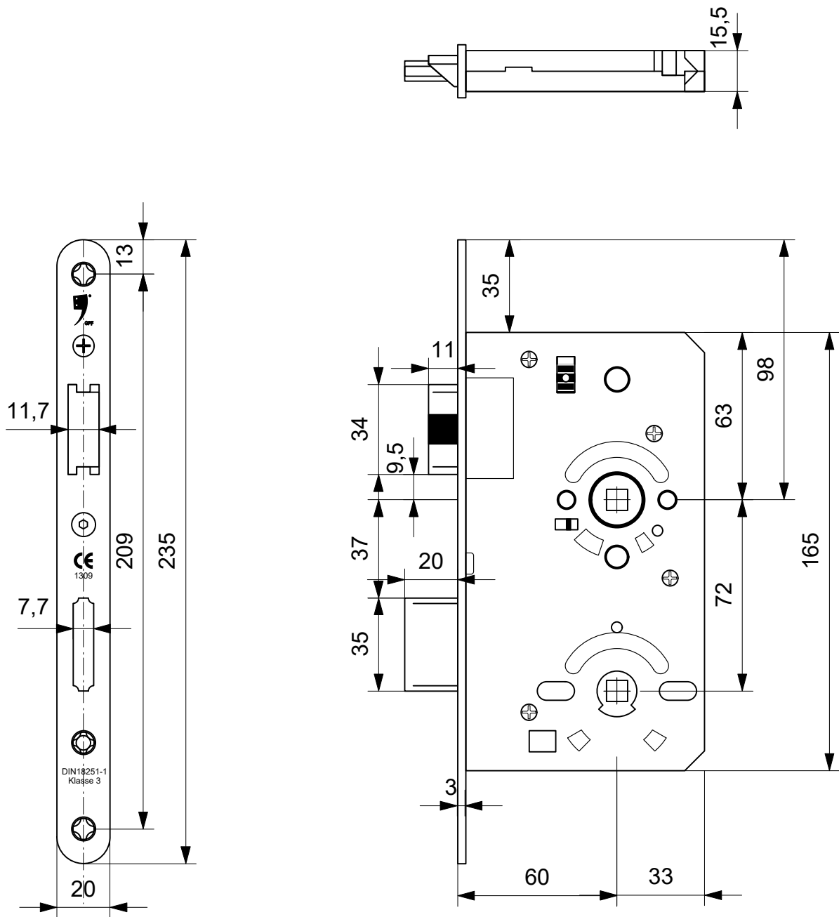
DIN links/rechts nastelbare gelagerde klemtuimelaar en fluisterdagschoot
